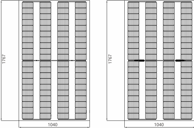
正面视图
